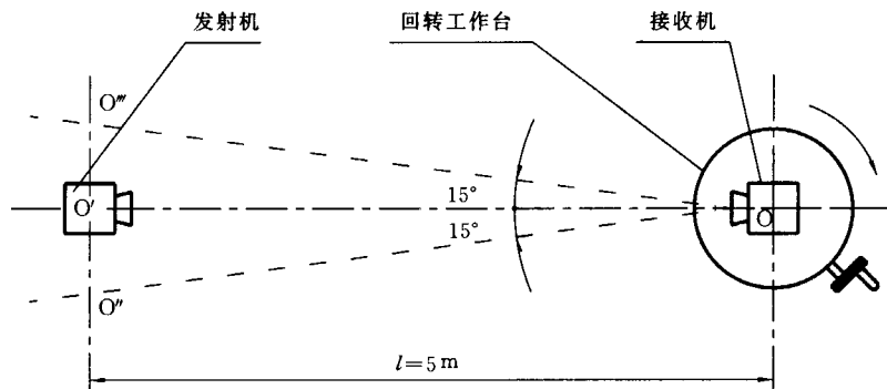
图2 接收机接收角度试验原理图
